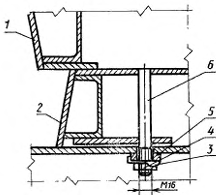
1 — шпиг; 2 — рамка; 3 — отгибная шайба, 4 — гайка; 5 — платик; 6 — шпилька
