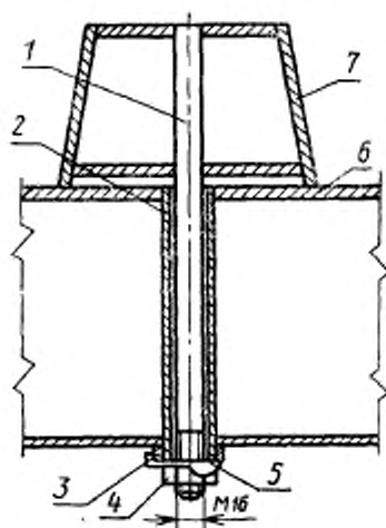
1 — шпилька; 2 — направляющая; 3 — пластик; 4 — гайка; 5 — отгибная шайба; 6 — поддон; 7 — вкладыш
