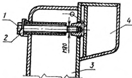
1 — болт; 2 — шайба отгибная; 3 — борт; 4 — вкладыш
