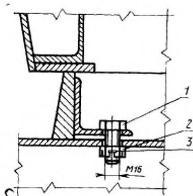
1 — болт; 2 — гайка; 3 — шпатель
