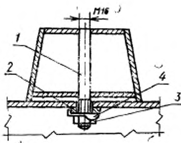
1 — шпилька; 2 — пластик; 3 — гайка; 4 — отгибная шайба
