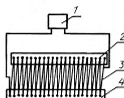
1 — записывающий прибор; 2 — термопары входного отверстия; 3 — соединительный провод; 4 — термопары выходного отверстия
