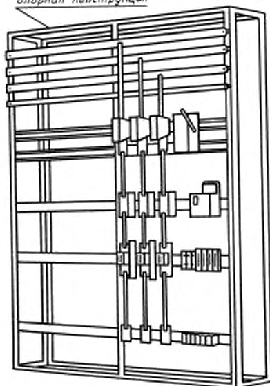
НКУ заводского изготовления открытого типа Черт. С.1
