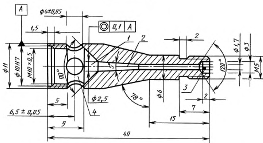
Трубка газовой горелки
