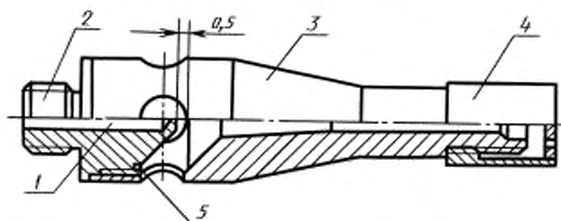
Конструкция газовой горелки
