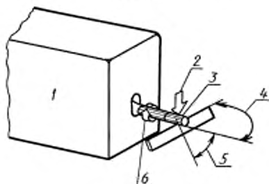
Устройство для определения остроты кромок
