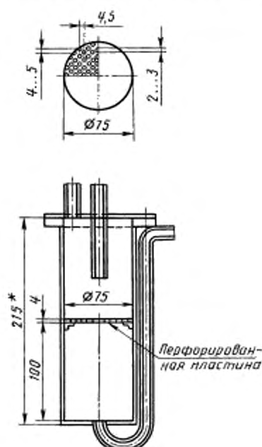
Комплект трубок для восстановления
