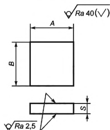
Рисунок А.1.7 — Контакт-деталь типа ПЦ
