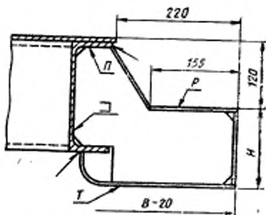
B —расстояние между направляющими поверхностями стоек пакетирушки; П —поверхность, взаимодействующая с крюком автоматического захвата; P —опорная поверхность для стойки автоматического захвата; T —поверхность, опирающаяся на кронштейн пакетирушки
