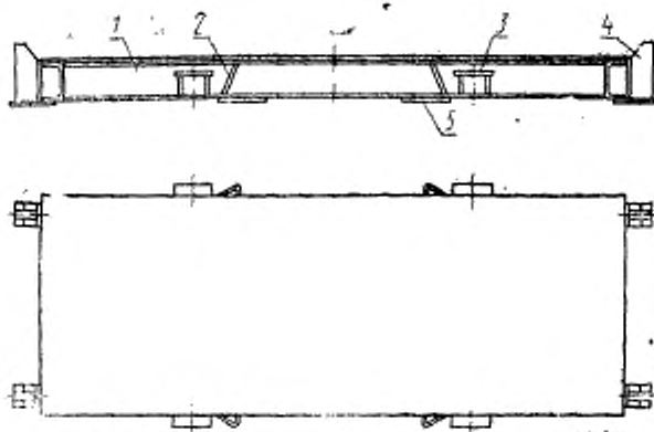
1—рама; 2—проушина; 3—кронштейн для автоматического захвата; 4—упор для натяжения арматуры; 5—плата для электромагнитного крепления формы к виброплощадке
