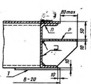
B —расстояние между направляющими поверхностями стоек пакетиروшки; П —поверхность, взаимодействующая с крюком автоматического захвата; P —опорная поверхность для стойки автоматического захвата; T —поверхность, опирающаяся на кронштейн пакетирушки
