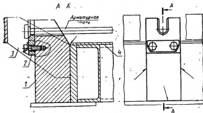
1—упор; 2—съемная пластина; 3—ограничение Черт. 1
