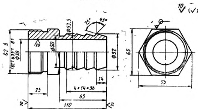
Штуцер Исполнение 1
