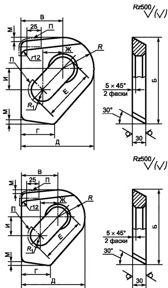
Рисунок Б.3 — Тип 2. Правое исполнение
