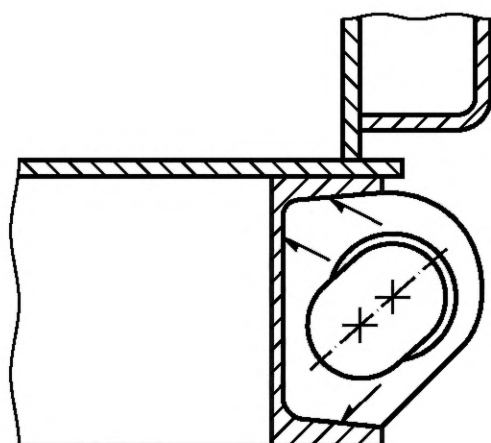
Рисунок Б.2 — Схема установки проушины. Тип 2
