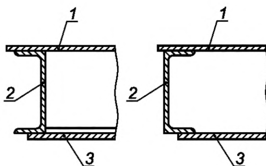
1 — настил (плоский или комбинированный); 2 — каркас; 3 — нижняя обшивка
