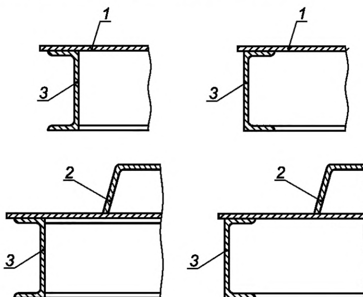
1 — плоский настил; 2 — комбинированный настил; 3 — каркас
