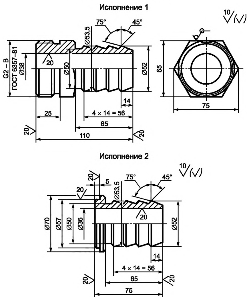
Рисунок А.1 — Штуцер
