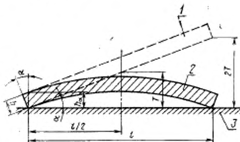
1 — мера с идеальной формой поверхности; 2 — реальная мера; 3 — базовая поверхность
