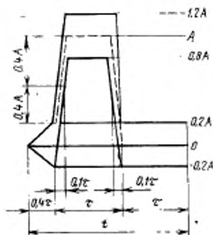
Трапецеидальный импульс ударной нагрузки
