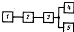
1 — генератор сигналов; 2 — согласующее устройство (эквивалент антенны); 3 — приемник; 4 — эквивалент нагрузки; 5 — вольтметр переменного тока
