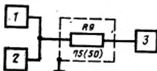
1 — генератор сигналов; 2 — универсальный вольтметр; 3 — приемник; R_0 — эквивалент антенны мощностью не менее 200 Вт
