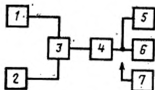
1 и 2 — генераторы сигналов; 3 — согласующее устройство (эквивалент антенны); 4 — приемник; 5 — эквивалент нагрузки; 6 — анализатор спектра; 7 — электронно-счетный частотомер
