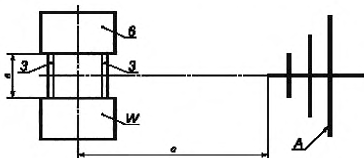
a = 1 м; А — измерительная антенна; W — оборудование для дуговой сварки с источником питания; 3 — сварочный провод (уложенный в петлю); Б — типовая нагрузка; с — расстояние в соответствии с ГОСТ 51317.4.3 и 6.3.3
