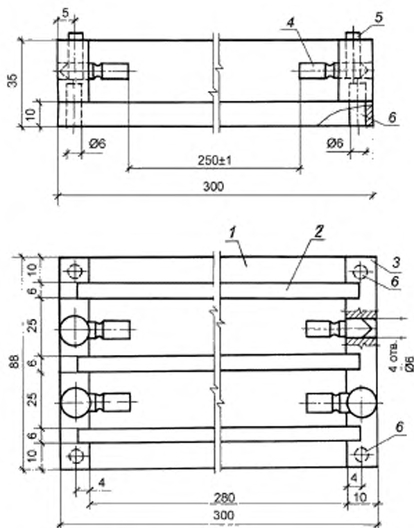
Рисунок В.1 — Форма для изготовления образцов-призм
