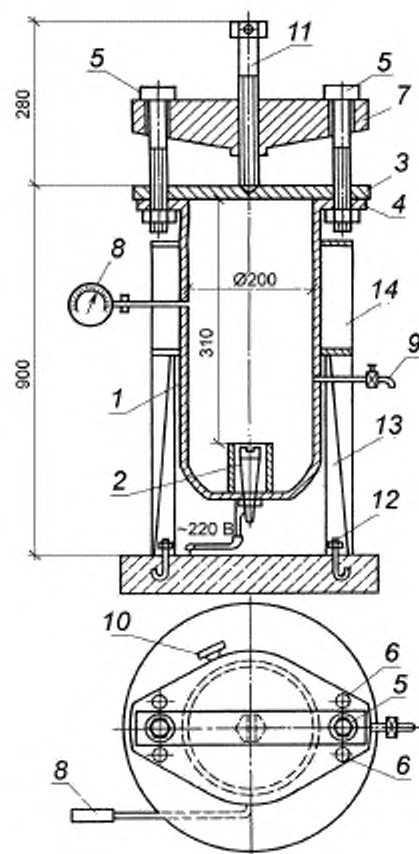
1 — корпус; 2 — нагревательные электроды; 3 — крышка; 4 — верхний фланец; 5 — бугельные болты; 6 — фланцевые болты; 7 — двухплечий бугель; 8 — электроконтактный манометр; 9 — кран для спуска пара и воздуха; 10 — предохранительный клапан; 11 — упорный винт; 12 — фундаментные болты; 13 — опоры; 14 — защитный кожух автоклава
