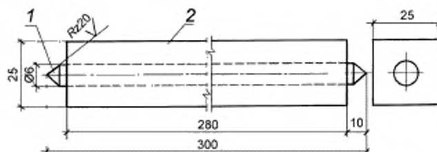
1 — стержень из нержавеющей стали; 2 — изолирующая оправа (дуб с последующим покрытием наружной поверхности лаком)
