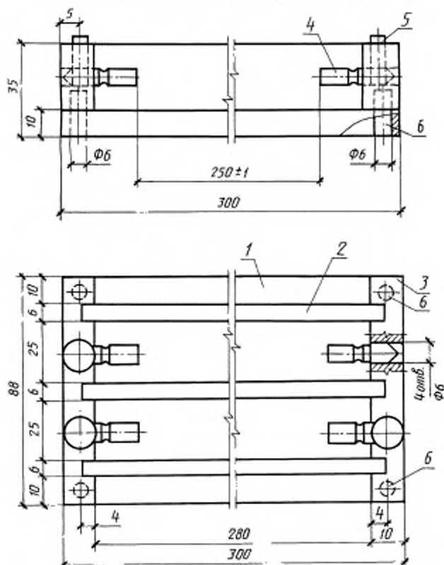
Форма для изготовления образцов-призм
