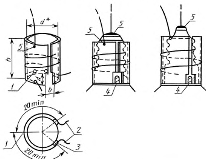
Испытательный патрон для цоколей E14/20 и E14/25 × 17
