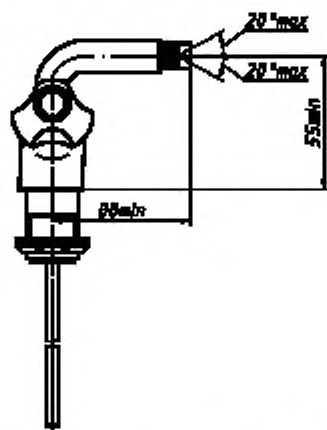
Рисунок 21 — Смеситель для бидвухрукояточный центральный напорный. Тип См-БдЦБ
