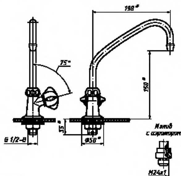
Рисунок 28 — Кран водоразборный напорный. Типы КрЦБр, КрЦБА
