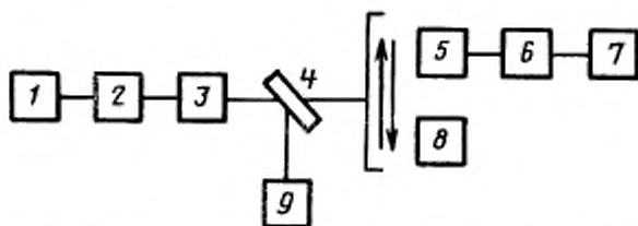
1 — лазер; 2 — модулятор; 3 — ослабитель; 4 — делительная пластина; 5 — первичный измерительный преобразователь исследуемого средства измерений; 6 — селективный усилитель; 7 — система регистрации; 8, 9 — контрольные средства измерений
