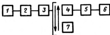
1 — светоизмерительная лампа с системой питания и контролем тока, 2 — модулятор, 3 — монохроматор; 4 — первичный измерительный преобразователь исследуемого средства измерений; 5 — селективный усилитель, 6 — система регистрации; 7 — контрольное средство измерений
