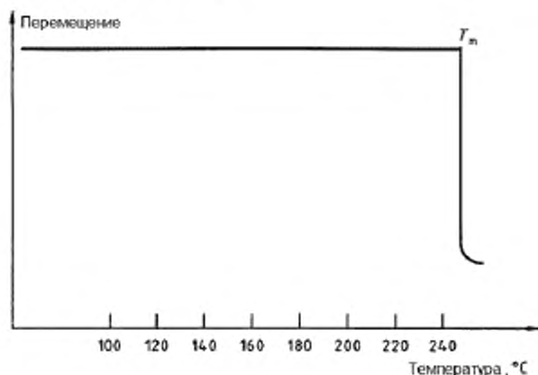
Рисунок 1 – Определение температуры плавления
