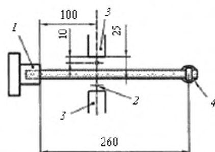
1 – крепление; 2 – термopар; 3 – горелка; 4 – груз Рисунок 17 – Вид испытательного устройства сверху
