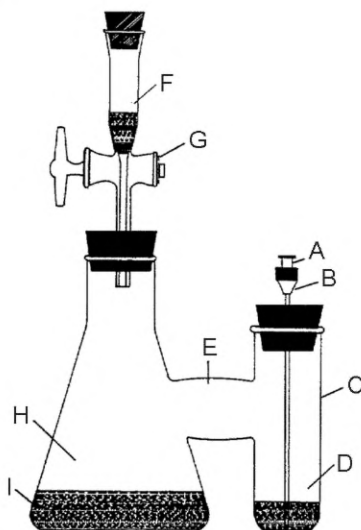
А — пробка из силиконовой резины; В — игла; С — пробирка; D — конец иглы, на которую надета силиконовая трубка; Е — соединяющий элемент между колбой Эрленмейера (Н) и пробиркой (С); F — фильтр с аскаритом; G — пробка с краном; Н — колба Эрленмейера; I — проба почвы
