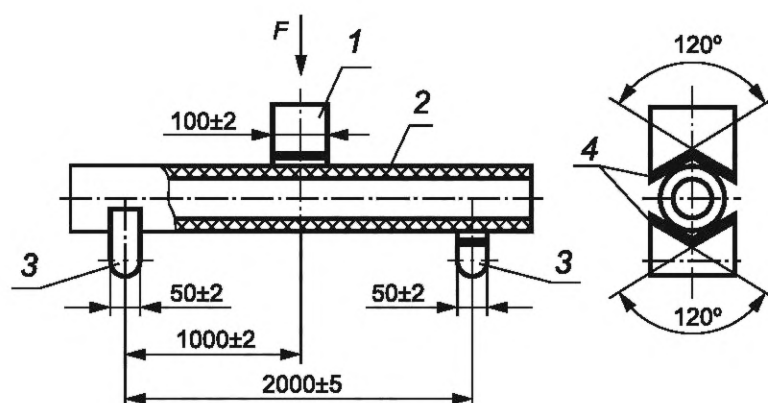
1 — деталь, передающая нагрузку; 2 — образец; 3 — опора; 4 — резиновая прокладка
