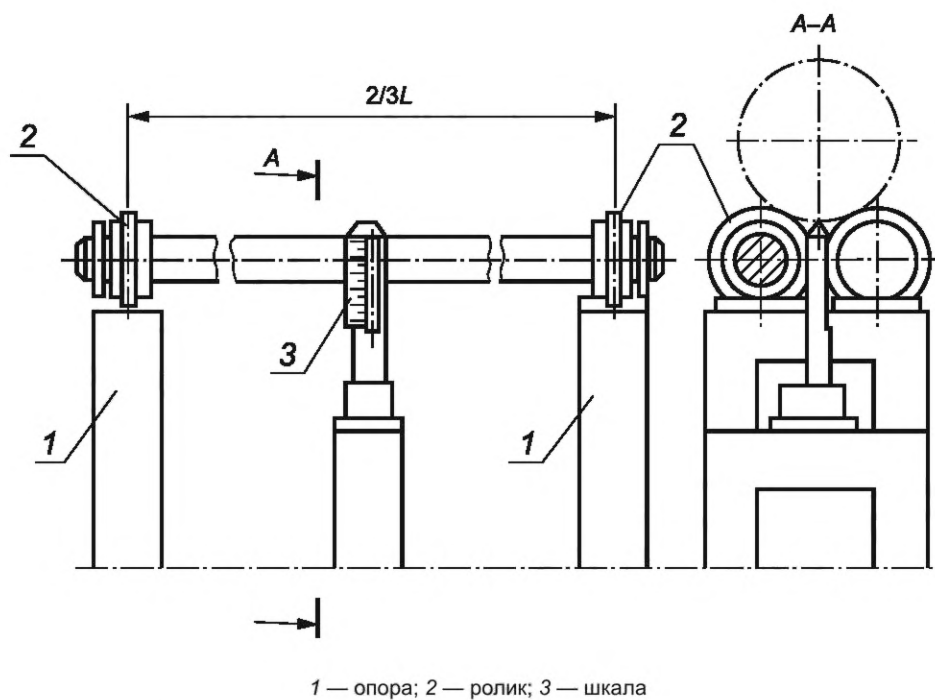
Рисунок А.1 — Схема станда для определения прямолинейности хризотилцементных труб
