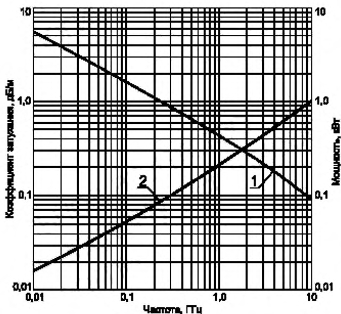
Частотные зависимости
