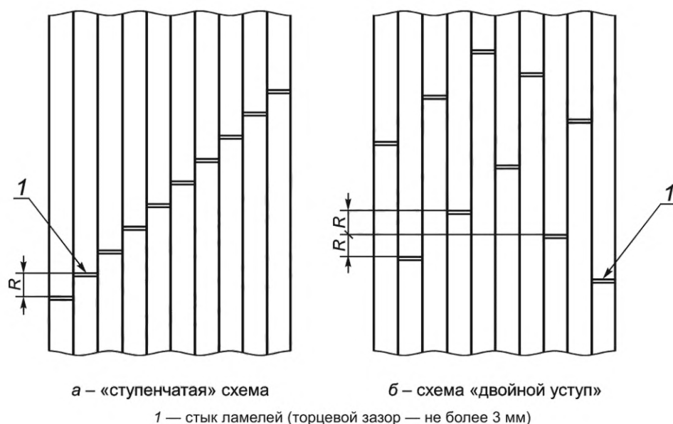
Рисунок 7 — Схемы укладки ламелей при сборке панелей
