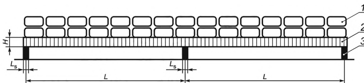
Рисунок В.3 — Расчетная схема нагружения двухпролетной панели
