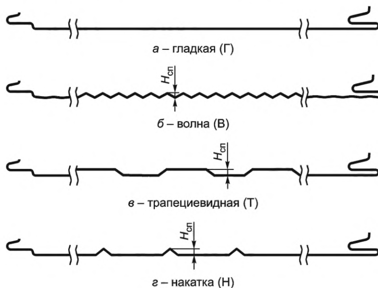
Рисунок 4 — Слабопрофилированные облицовки
