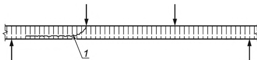
Рисунок А.4 — Схема испытания образца на поперечный изгиб
