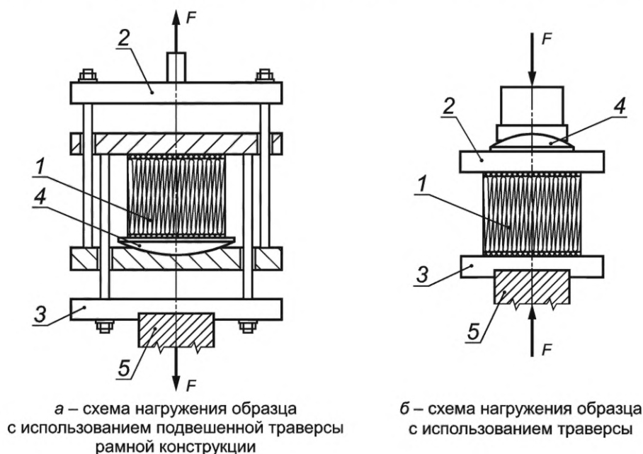
1 — испытуемый образец; 2 — верхняя траверса испытательной машины; 3 — нижняя траверса; 4 — шарнирная опора; 5 — рама машины
