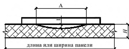
Рисунок 16 – Схема измерения отклонения от плоскостности
