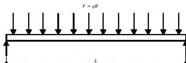
Рисунок Б.3 – Воздействие воздушного давления или вакуума
