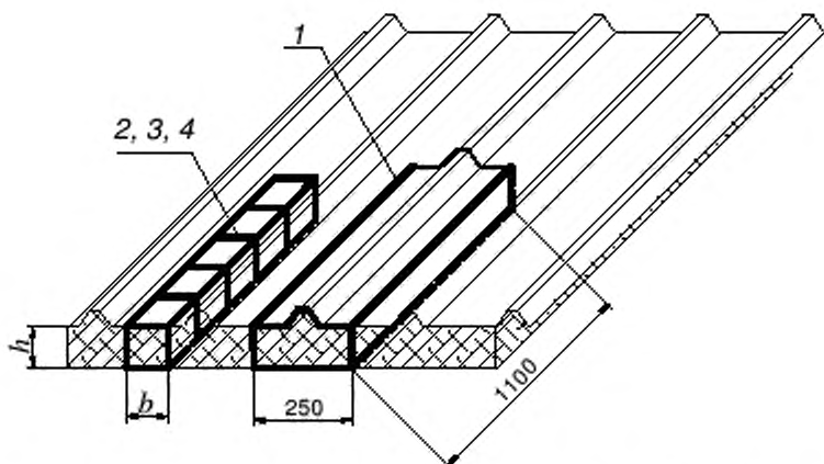
1 — зона вырезки образца для испытаний прочности на поперечный изгиб; 2 — зона вырезки образца для испытаний прочности на сжатие; 3 — зона вырезки образца для испытания прочности на растяжение; 4 — зона вырезки образца для определения физических свойств сердцевины (объемная масса, влаго- и водопоглощение, теплопроводность и др.)
