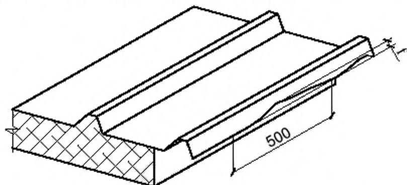
Рисунок 17 – Схема измерения отклонения кромки свободного гофра стыка
