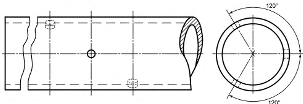
Рисунок Г.1 — Эталонный образец с тремя отверстиями
