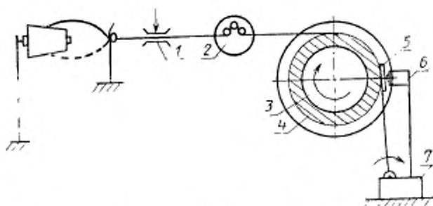
1—тарельчатый натяжитель; 2—тензиометр для измерения натяжения нити; 3—катушка для наматывания нити до постоянного объема; 4—наматываемый слой нити; 5—контактная пластинка для контроля высоты наматываемого слоя нити; 6—ограничитель контактной пластинки; 7—приспособление для останова двигателя
