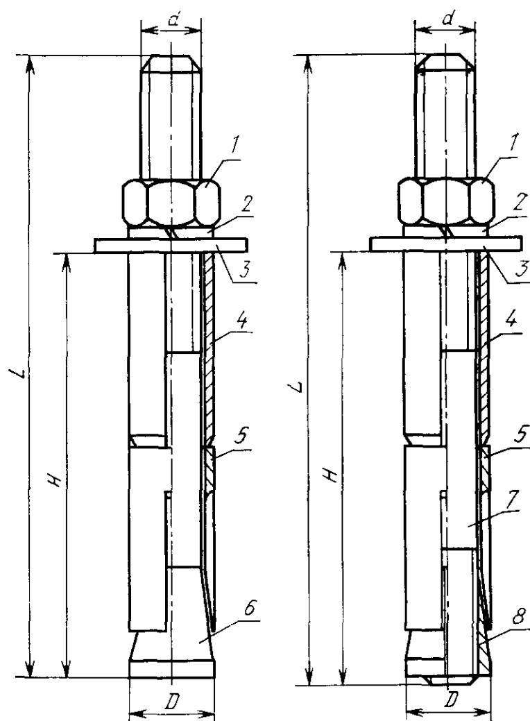
Исполнение 1
