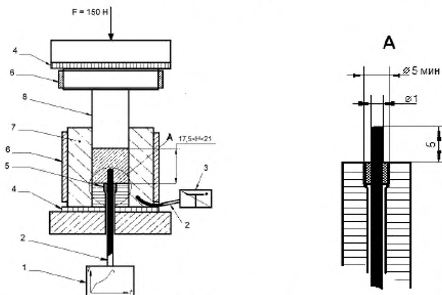
1 – температурное записывающее устройство, 2 – термозлемент, 3 – система контроля температуры, 4 – изоляция, 5 – изоляция термозлемента, 6 – нагревательный прибор, 7 – цилиндрическая форма, 8 – нагретый стальной пуансон.
