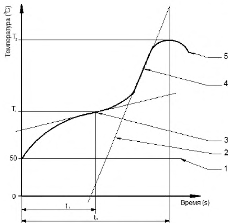
1 – измерение начальной температуры, 2 – угол наклона к линии зависимости температуры от времени во второй точке перегиба, 3 – первая точка перегиба, 4 – вторая точка перегиба, 5 – остановка записи.
