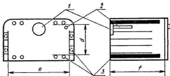
1—дверца жарочного шкафа; 2—ручка терморегулятора; 3—нагревательные элементы
