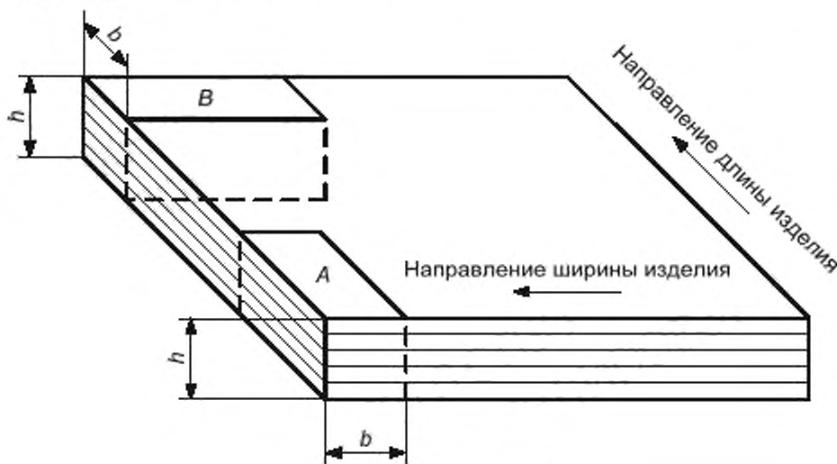
Рисунок 3 – Расположение образцов
