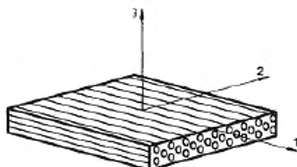
Рисунок 1 — Элемент пластины из композиционного материала, армированного однонаправленным волокном с указанием осей симметрии
