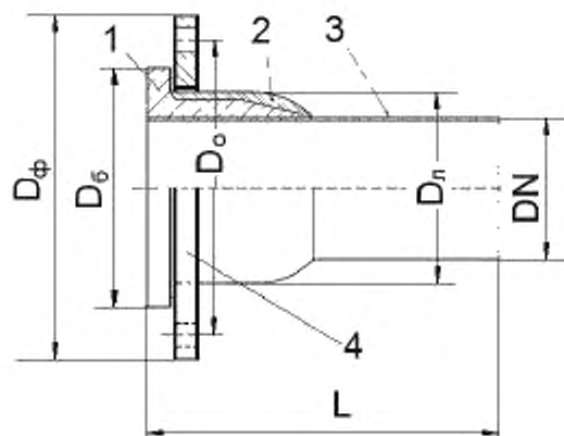
1 – формованный упорный буртик; 2 – ламинирование буртика и патрубка; 3 – фланцевый патрубок; 4 – накладное стальное кольцо; D б – диаметр упорного буртика
