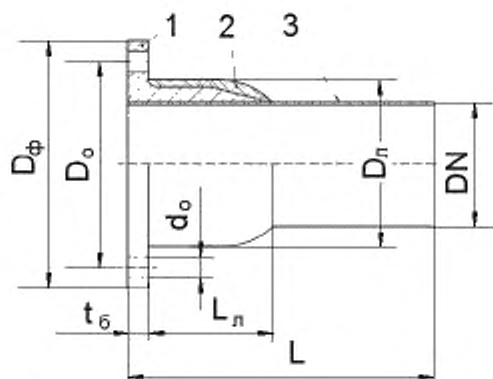
1 – формованный фланцевый буртик; 2 – ламинирование буртика и патрубка; 3 – фланцевый патрубок; L – длина фланца; L л – длина ламинирования; t б – толщина буртика; D о – диаметр окружности по присоединительным отверстиям; d о – диаметр присоединительных отверстий; D н – диаметр ламинированной части патрубка; D ф – диаметр фланца
