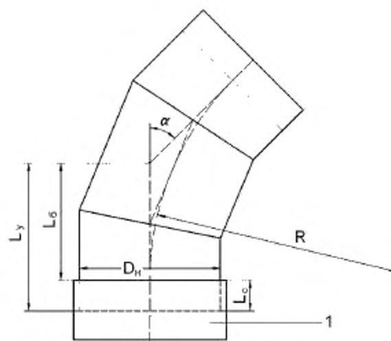
1 – муфта; D_n – наружный диаметр трубы; L_y – уложенная длина отвода; L_б – базовая длина; L_с – длина соединения; \alpha – угол отвода; R – радиус отвода.
