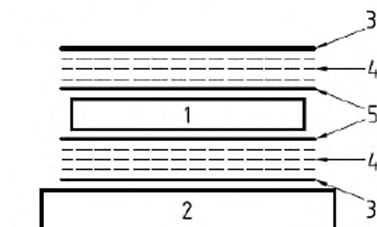
1 – образец для испытаний; 2 – рабочая поверхность; 3 – непористая антиадгезионная пленка; 4 – впитывающая стеклоткань (три слоя); 5 – антиадгезионная перфорированная пленка
