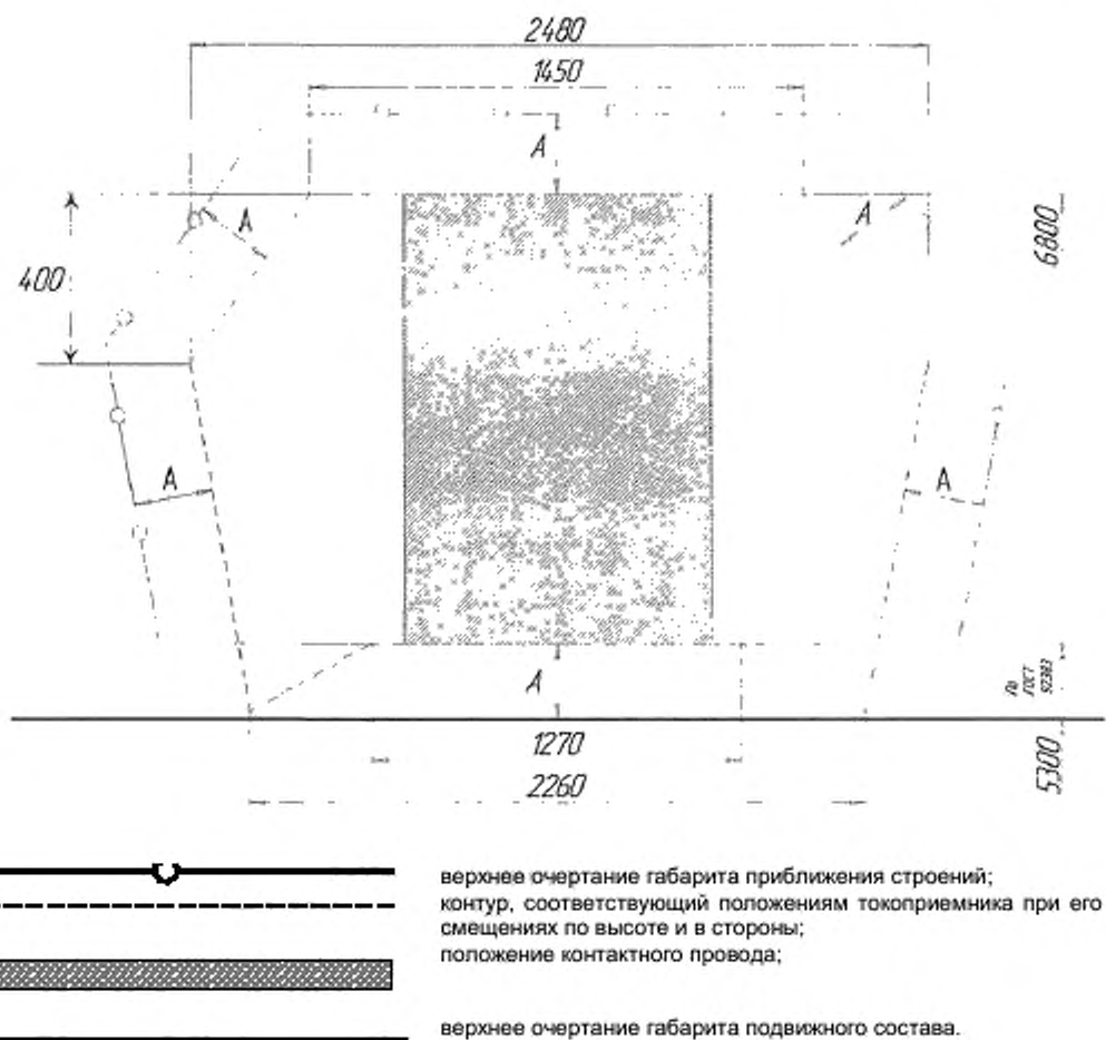
Рисунок 1 — Расстояния между сооружениями, устройствами контактной сети, токоприемниками и подвижным составом
