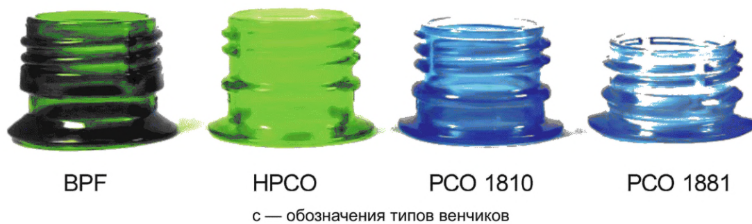
Рисунок Б.2 — Типы венчиков горловин преформ
