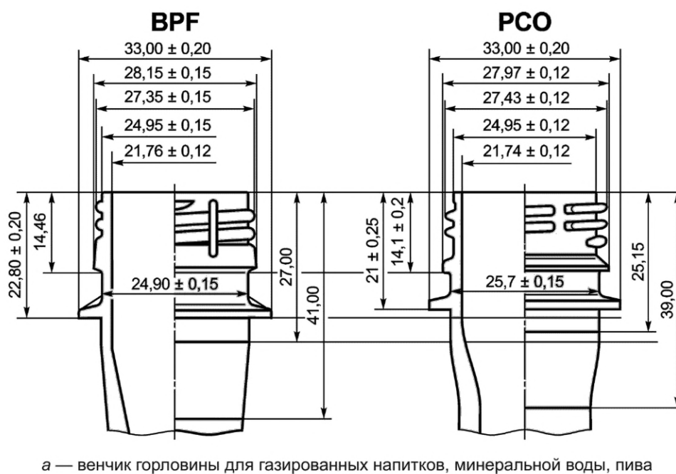
Рисунок Б.1 — Типы преформ
