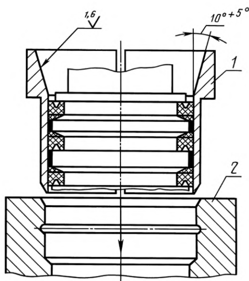
1 — оправка; 2 — цилиндр
