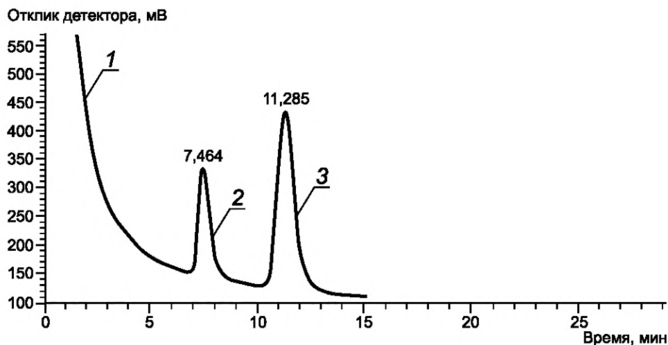
Рисунок 1 — Хроматограмма определения антиоксиданта агидола-2
