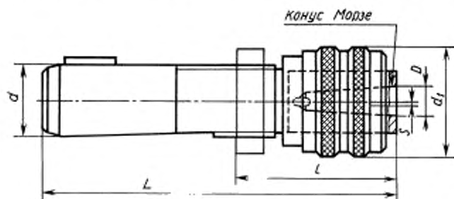
Размеры, мм
