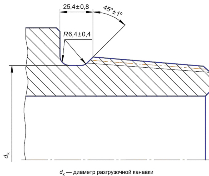
Рисунок 6 — Разгрузочная канавка на ниппельном конце
