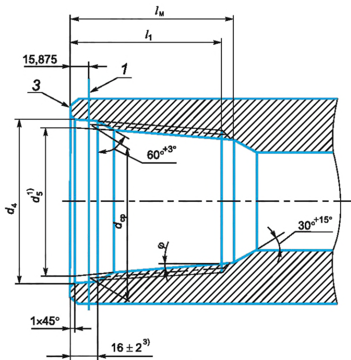
б — Муфтовый конец»;
