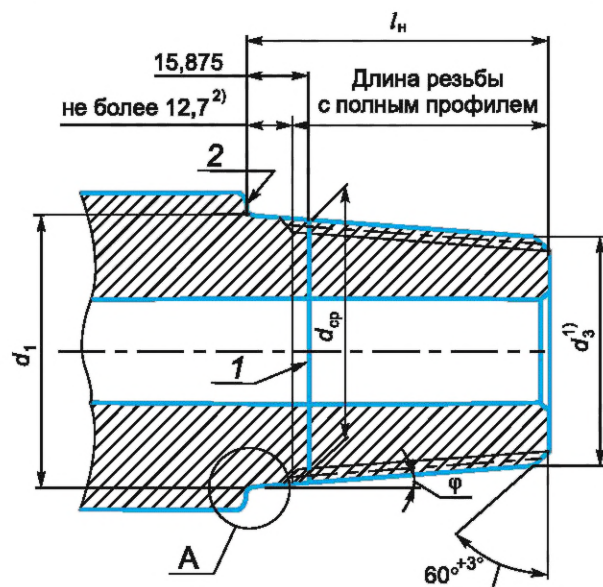
а — Ниппельный конец
