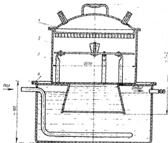
1—крышка; 2—корпус; 3—подставка с отверстиями для фильтров; 4—подогревающая баня
