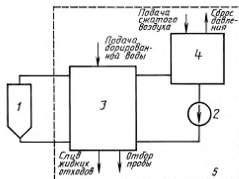
Структурная схема стенда КГО
