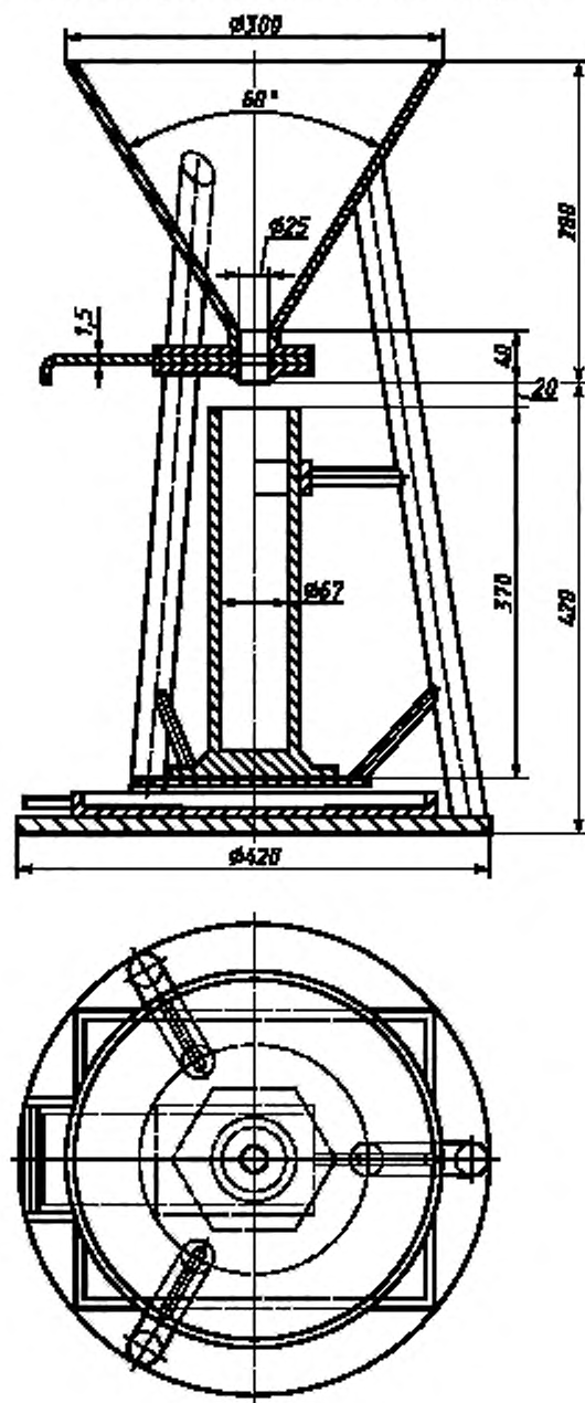
Аппарат для определения насыпной плотности удобрений
