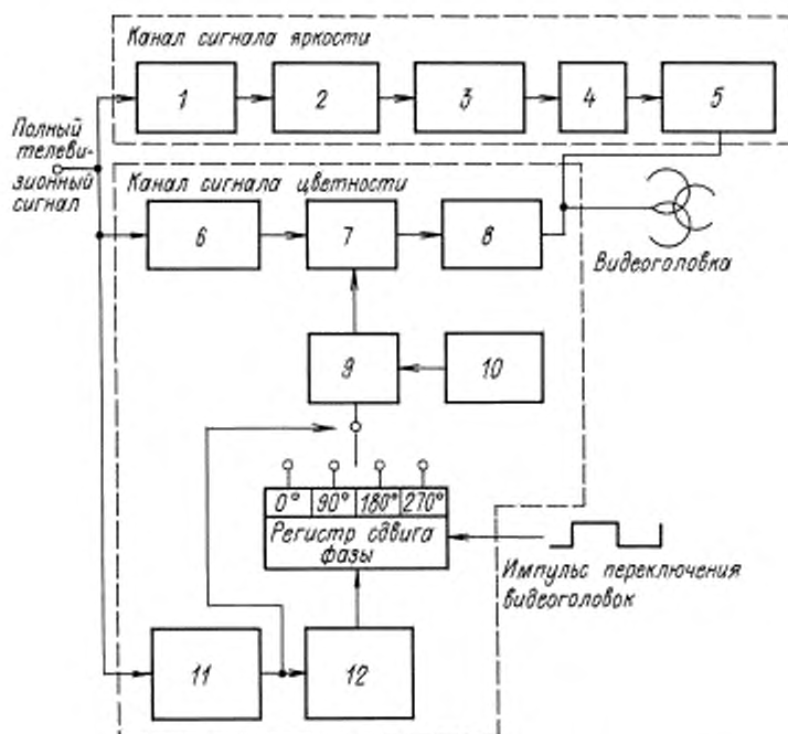
1, 8 — фильтры нижних частот; 2 — схема частотных предискажений; 3 — частотный модулятор; 4 — фильтр верхних частот; 5 — усилитель записи; 6 — полосовой фильтр; 7, 9 — преобразователь частоты; 10 — гетеродин; 11 — схема выделения сигналов строчной синхронизации; 12 — умножитель частоты
