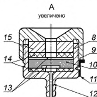
Рисунок А.1 — Схема гидродинамического прибора
