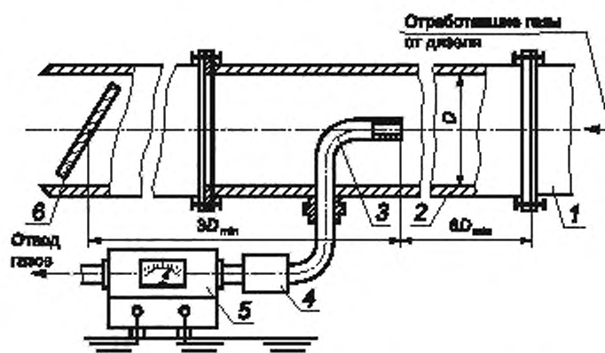
1 — выпускной трубопровод дизеля; 2 — выпускная труба испытательного стенда; 3 — газоотборник дымометра; 4 — ресивер; 5 — измерительный прибор; 6 — регулирующая заслонка
