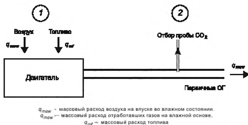
Рисунок 4 — Точки замера для проверки расхода углерода
