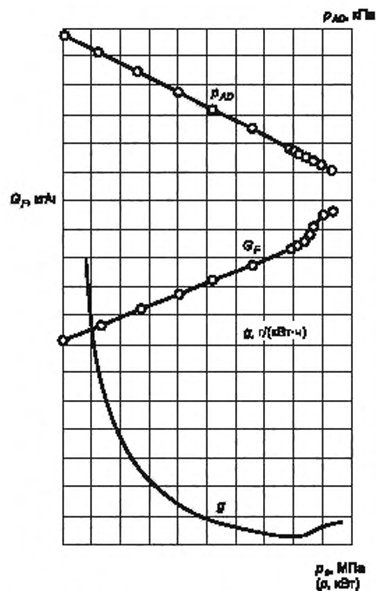
Рисунок Е.5 — Нагрузочная характеристика двигателя
