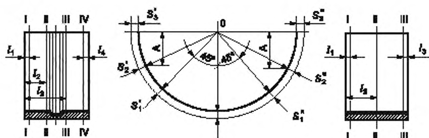
а) Вкладыши с кольцевой масляной канавкой
