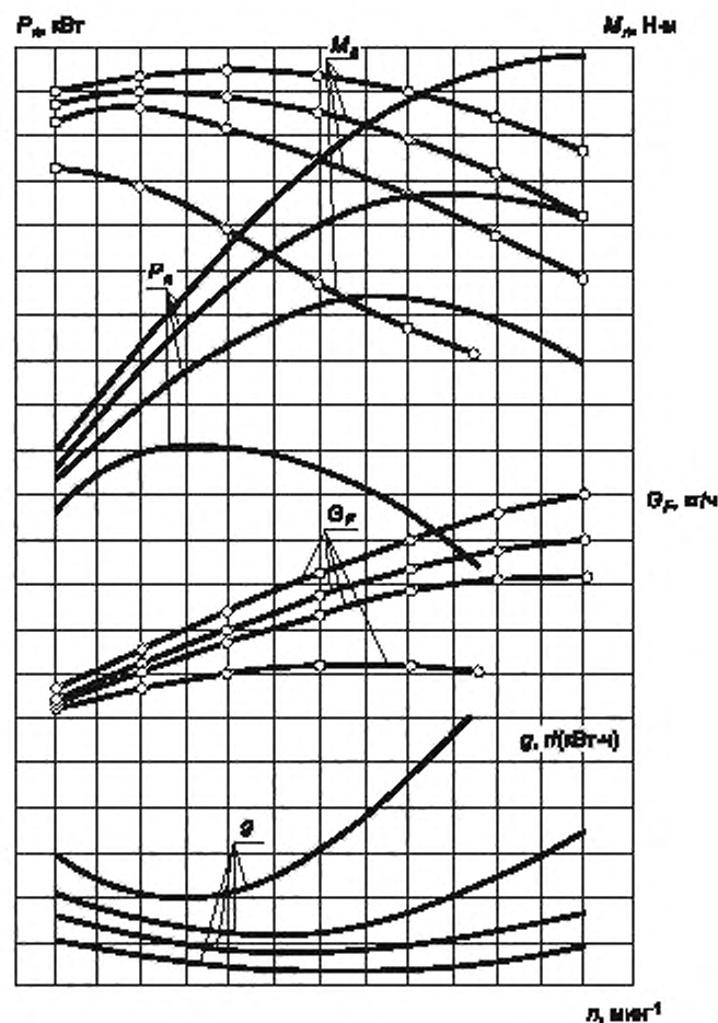
Рисунок Е.3 — Скоростные частичные характеристики двигателя (при различных положениях дроссельной заслонки)
