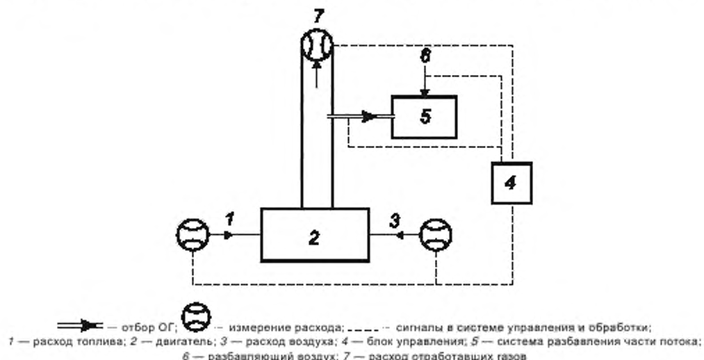
Рисунок 1 — Схема измерения выбросов взвешенных частиц с использованием туннеля для разбавления части потока ОГ
