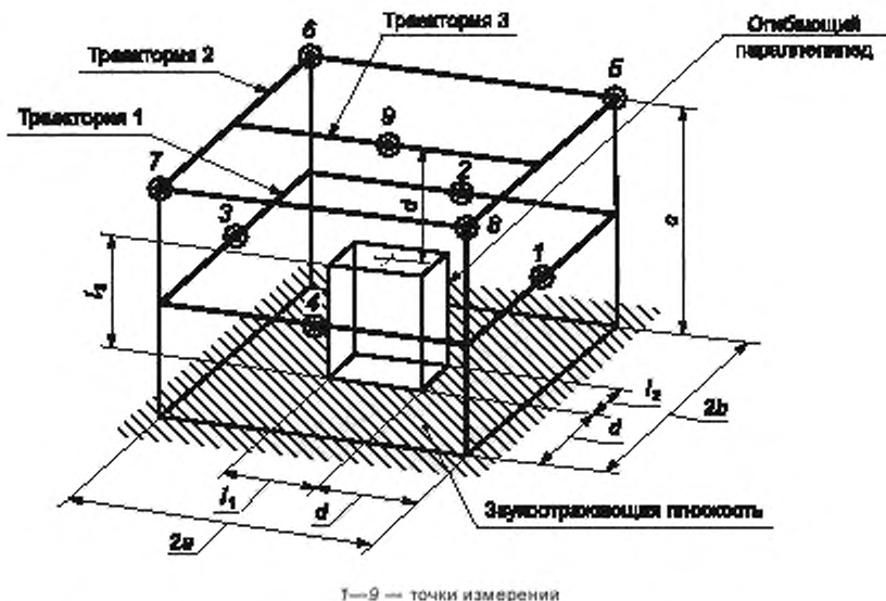
Рисунок Ж.1 — Пример измерительной поверхности и положений (траекторий) микрофонов
