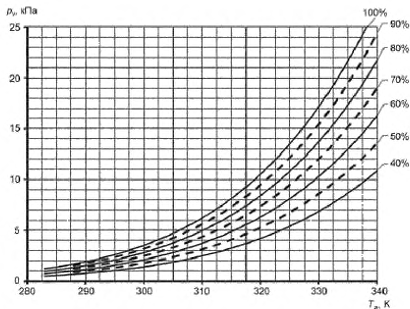
Рисунок Л.1 — График зависимости парциального давления водяного пара p_v от температуры и относительной влажности воздуха
