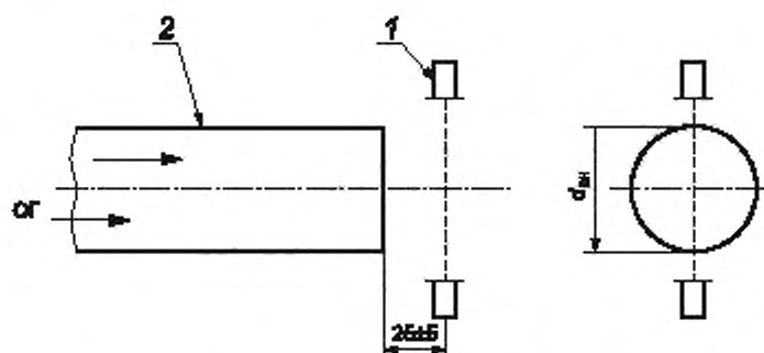
1 — полнопоточный дымометр; 2 — выпускная труба круглого сечения, ОГ — поток ОГ; d_{\text{вн}} — внутренний диаметр выпускной трубы ( d_{\text{вн}} может быть приравнен к наружному диаметру выпускной трубы при толщине стенок менее 1,5 мм)
