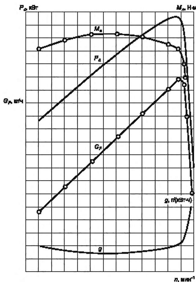
Рисунок Е.2 — Скоростная характеристика с регуляторной ветвью двигателя
