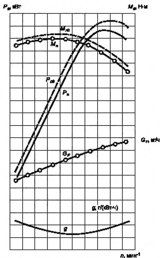
Рисунок Е.1 — Внешняя скоростная характеристика (ВСХ) двигателя
