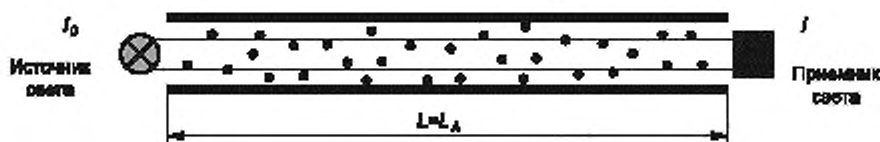
Рисунок Д.1 — Схема прибора для измерения дымности
