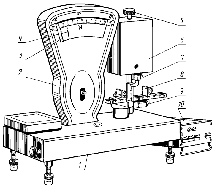
ПРИБОР ИБ 5058—0,04
