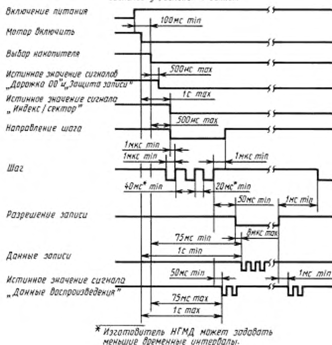
Требования к основным временным соотношениям сигналов управления и данных
