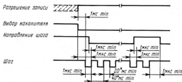
Временная диаграмма доступа к дорожке
