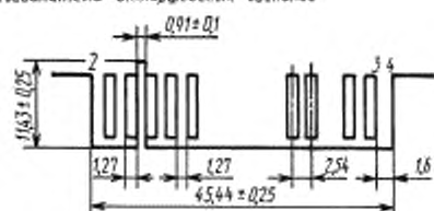
Соединитель интерфейсных сигналов
