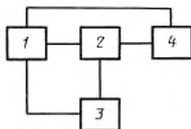
1 — формирователь обрабатываемого сигнала; 2 — измеряемое изделие; 3 — индикатор сигнала на выходе конвольвера; 4 — формирователь опорного сигнала
