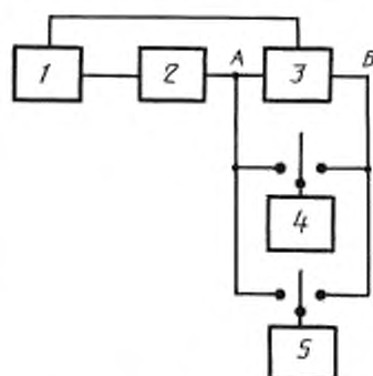
1 — генератор коротких радиопульсов с прямоугольным спектром; 2 — измеряемое изделие; 3 — устройство стробирования импульсов; 4 — анализатор спектра; 5 — измеритель структуры импульсного отклика
