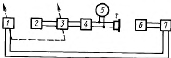
1 — регистрирующее устройство; 2 — генератор розового шума ГШН; 3 — узкополосный фильтр; 4 — усилитель мощности УМ; 5 — вольтметр; 6 — камера связи; 7 — микрофонный измерительный усилитель УИМ; Т — телефон
