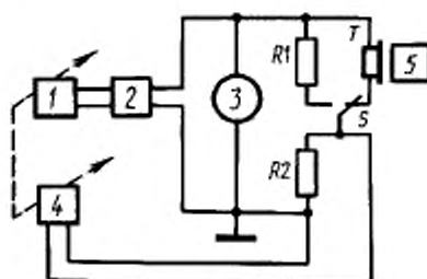
1 — генератор ГСН; 2 — усилитель мощности У1; 3 — вольтметр; 4 — регистрирующее устройство; 5 — камера связи; R1 — резистор или магазин сопротивлений; R2 — резистор; T — телефон; S — переключатель
