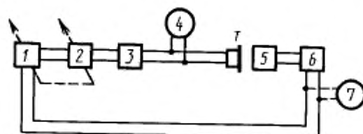
1 — регистрирующее устройство; 2 — генератор ГСН; 3 — усилитель мощности У1; 4 — вольтметр; 5 — камера связи; 6 — микрофонный измерительный усилитель УИМ; 7 — вольтметр
