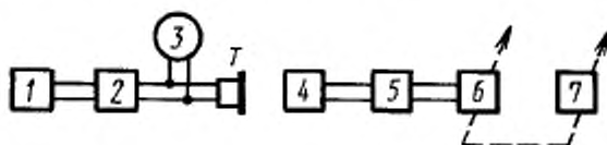
1 — генератор розового шума ГШН; 2 — усилитель УМ; 3 — вольтметр; 4 — камера связи; 5 — микрофонный измерительный усилитель УИМ; 6 — переключаемый узкополосный фильтр; 7 — регистрирующее устройство; Т — телефон
