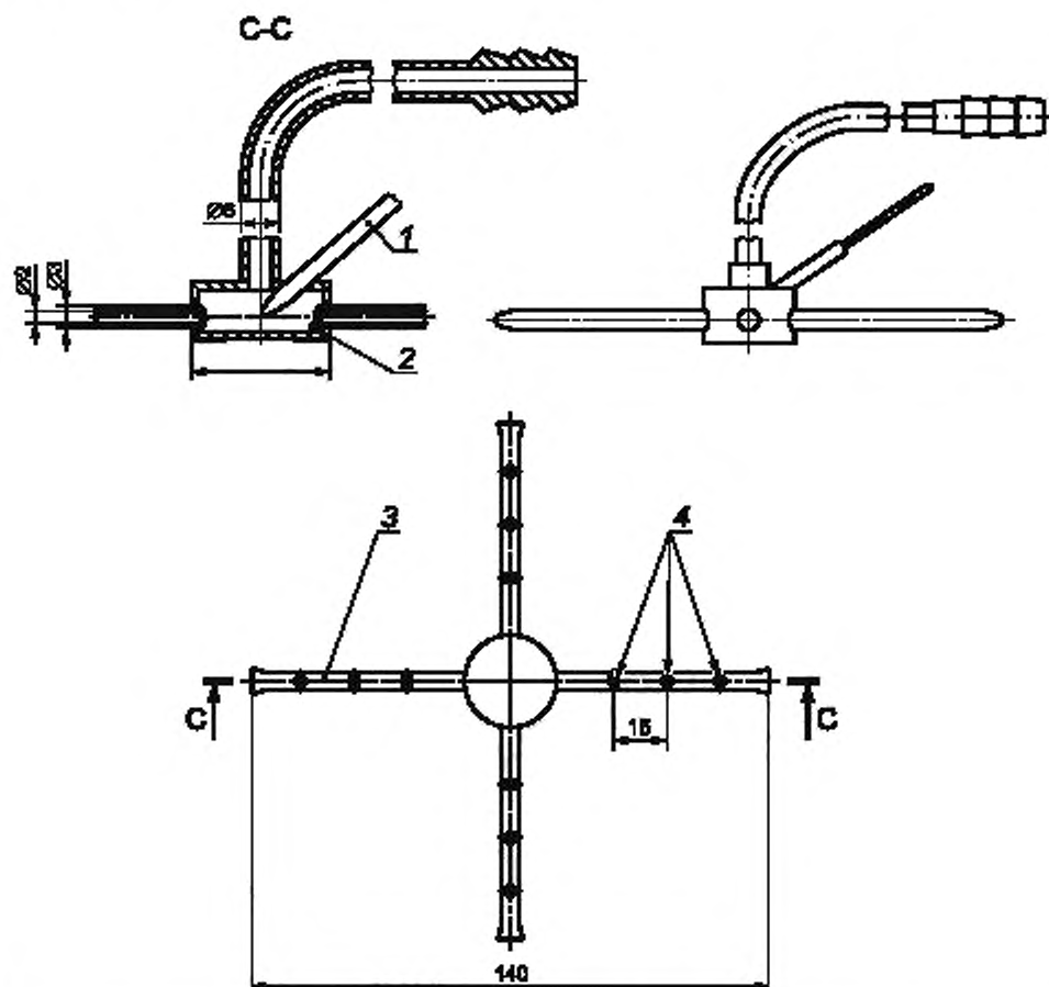
1 — трубка с двумя каналами, в которых расположены провода термодатчиков; 2 — точка измерения температуры; 3 — трубка с глухим концом; 4 — отверстия
