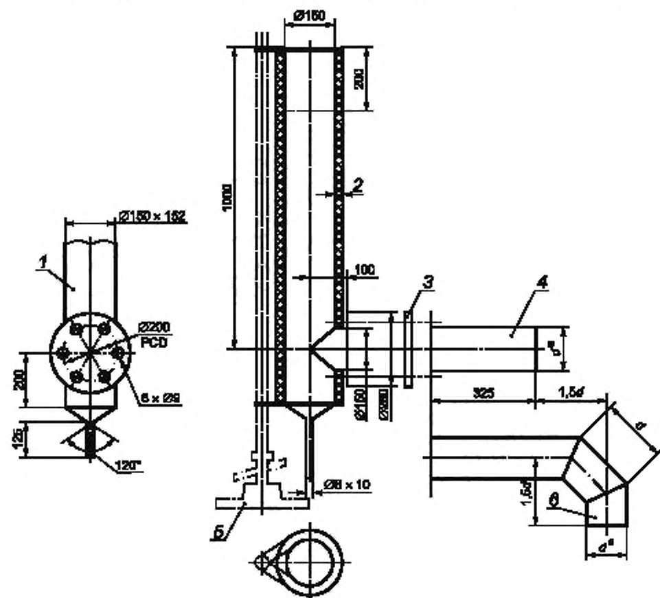
1 — труба дымохода из нержавеющей стали; 2 — теплоизоляция (стекловолно плотностью 64 \text{ кг/м}^3 ); 3 — прокладка; 4 — соединительная труба из нержавеющей стали; 5 — опорная стойка; 6 — соединительная труба из нержавеющей стали
