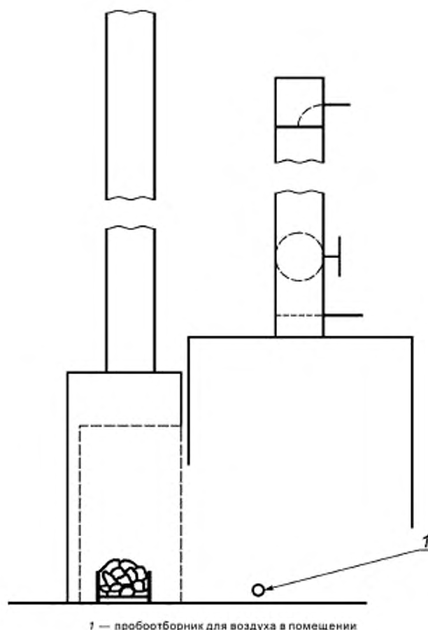
Рисунок 2 — Вытяжной зонд
