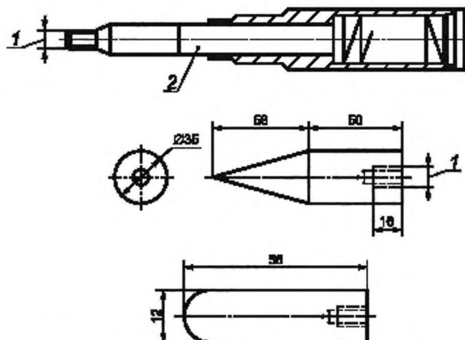
1 — диаметр 6 мм; 2 — устройство, создающее усилие 5 Н, с двумя шкалами, для вертикальной и горизонтальной плоскости измерения
