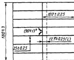
Испытательная панель с прорезями
