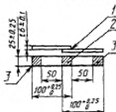
Образец для испытаний
