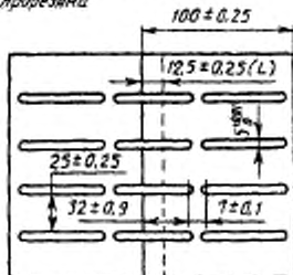
Испытательная панель с прорезями
